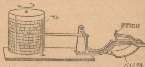
第20図 自記温度計
