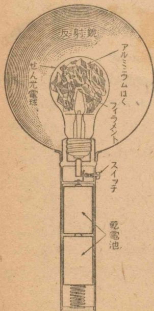
第10図 セン光電球
