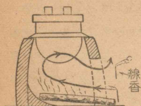
第25図 かまど (1)
