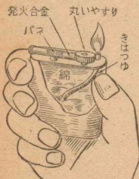
第44図 ライターの構造
