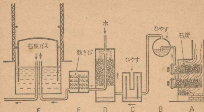
第16図 石炭ガスができるまで
