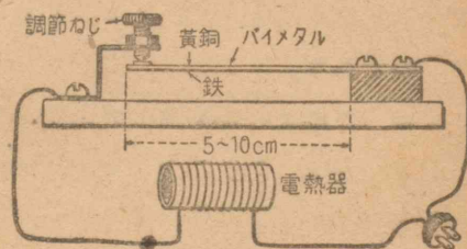
第21図 サーモスタット
