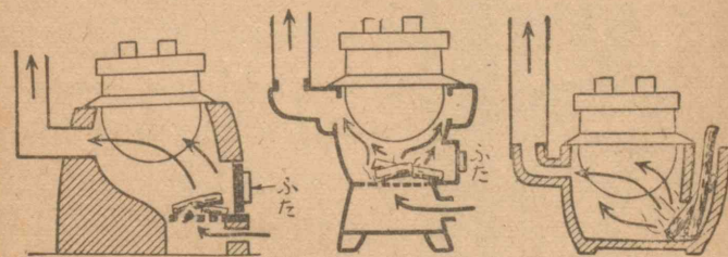
第32図 いろいろなかまど(5)
