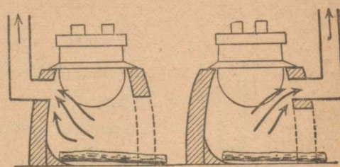
第31図 かまど(4)
