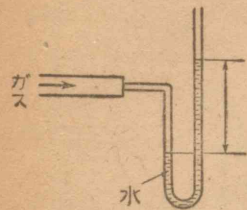
第33図 マノメーター
