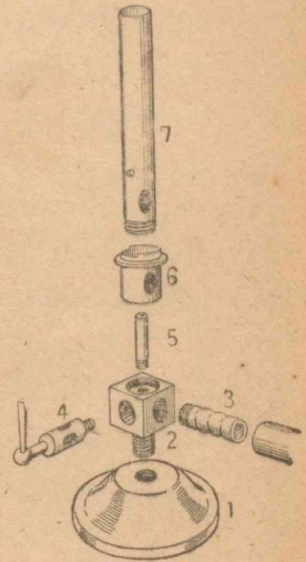
第35図 ガスバーナー
