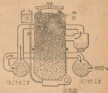
第3図 乗合自動車の木炭ガス発生炉
