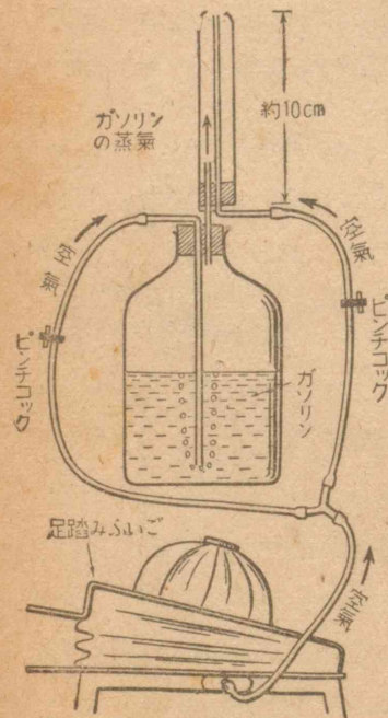
第 38 図 エアガス装置
