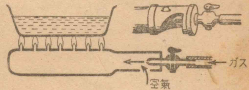
第37図 ガスコンロ
