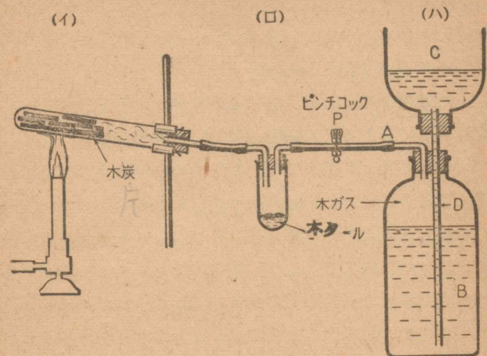
第 13 図 実験 9. のしかけ
