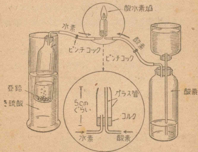
第 40 図 実験 14. 酸素水素えん
