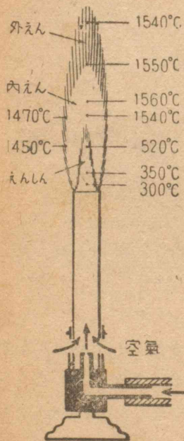
第36図 バーナーのほのお
