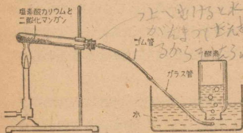
第 8 図 実験 7. の装置
