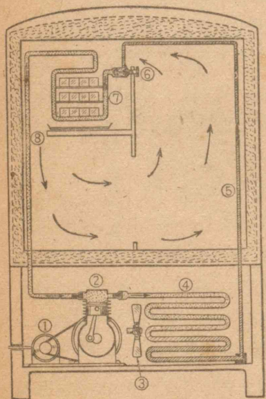
第 51 図 電気冷蔵庫
