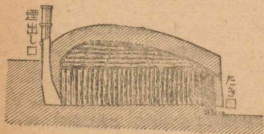
第15図 炭焼きがま
