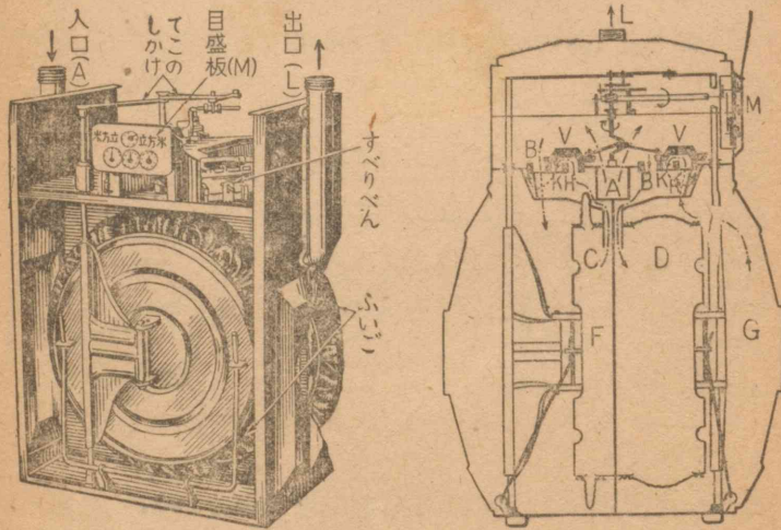
(1) 第34図 ガスメートル (2)
