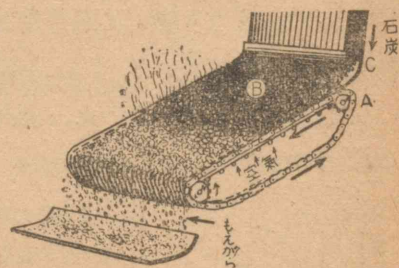
第29図 ストーカ
