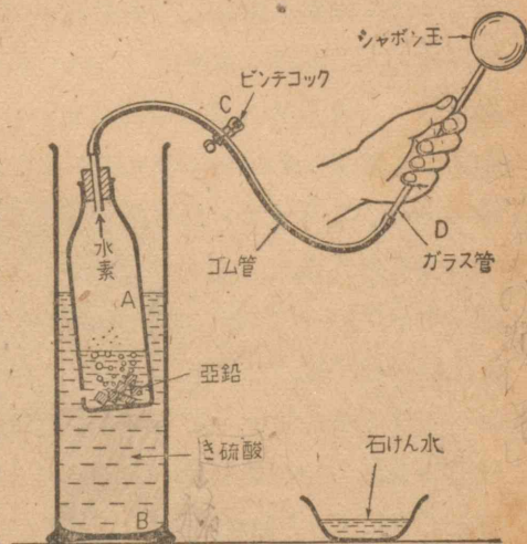
第4図 実験4.の装置
