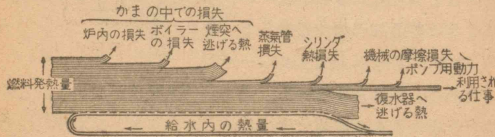
第115図 蒸気機関の熱の行くえ
