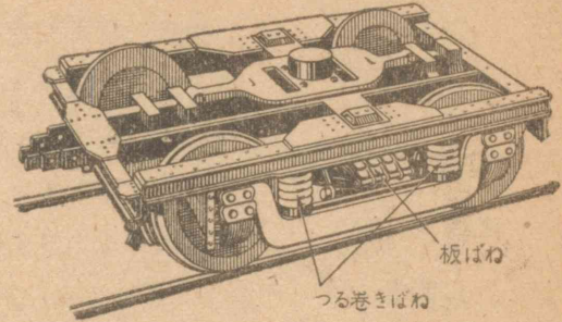
第 38 図 電車車輪部
