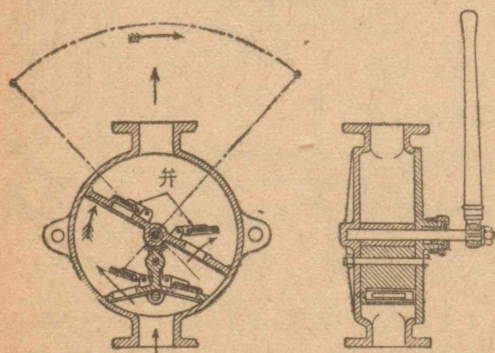
第 92 図 ウィングポンプ
