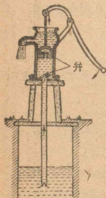
第 91 図 吸上げポンプ のすき間
