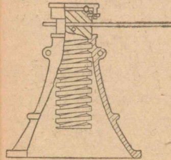
第53図 ジャッキ
