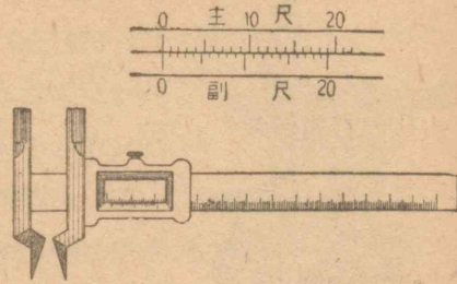
第 61 図 ノギスと副尺
