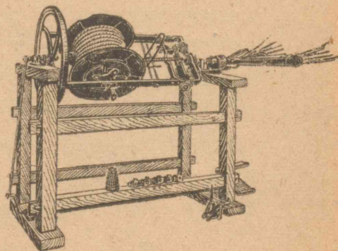
第9図 足踏みなわない機
