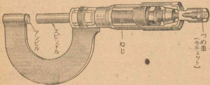
第58図 ねじ測微計
