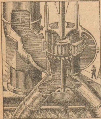
第102図 フランシス水車
