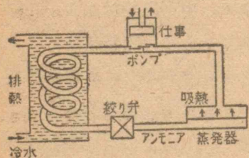
第121図 冷凍機の原理
