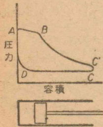
第116図 指圧線図 シリンダ内の気圧と容積の関係を示す。
