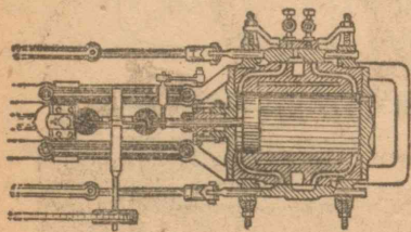
第123図 ルノアールのガス機関
