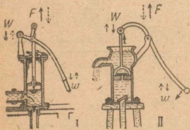
第 26 図 (b) ポンプの柄
