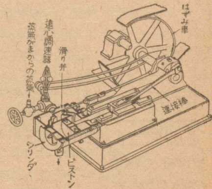
第114図 蒸気機関
