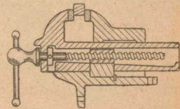
第55図 万力
