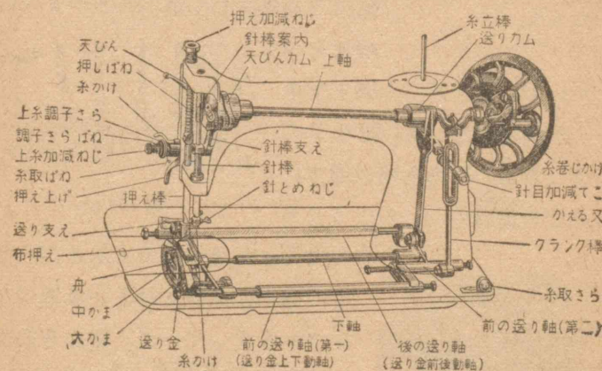
第107図 ミシン
