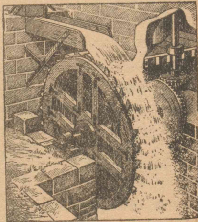
第106図 上掛け水車
