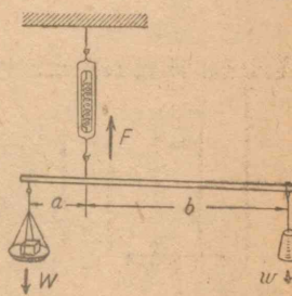
第 25 図 さおばかりの
