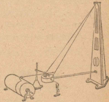
第43図 地震計(水平動)
