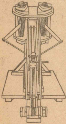
第 36 図 石投機
