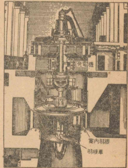
第103図 カプラン(プロペラ)水車
