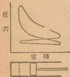
第124図 内燃機関指圧線図
