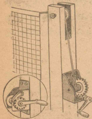
第 20 図 ネットを張る機械
