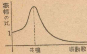
第40図 共振曲線
