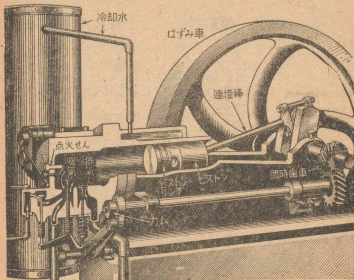
第126図 オットーのガス機関 オットーは混合ガスを吸いこんでそれを圧縮し、つぎに爆発させ最後に排気するという4行程を行わせ、その中の1行程で動力を得るようにした。なお調整歯車にはねじ歯車を使った。
