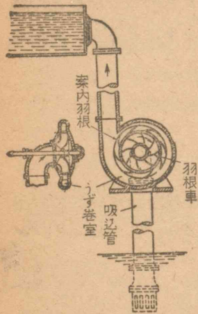
第96図(a) うず巻ポンプ
