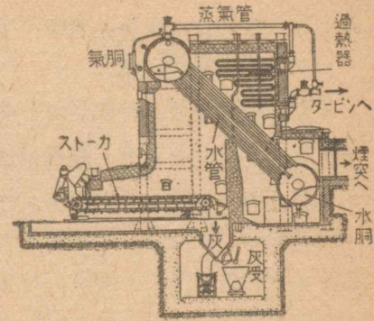
第117図 蒸気がま
