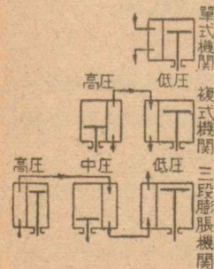
第118図 多段膨脹機関
