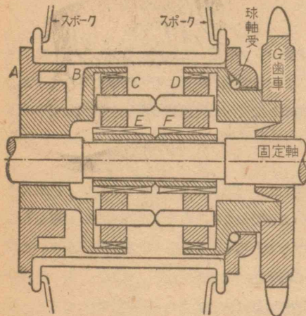
第76図 増速比変換装置の一例
