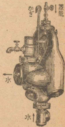
第97図 だるまポンプ ときりのよな器が2箇あり、交互に水を吸いこみ蒸気で押し上げる。かぎは使うときに上からつすためのものである。
