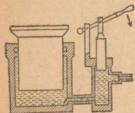
第98図 水圧機
