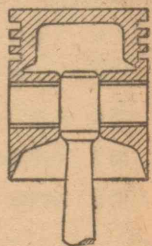
第126図 オットーのガス機関 オットーは混合ガスを吸いこんでそれを圧縮し、つぎに爆発させ最後に排気するという4行程を行わせ、その中の1行程で動力を得るようにした。なお調整歯車にはねじ歯車を使った。
