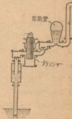
第95図 ブランジャーポンプ
