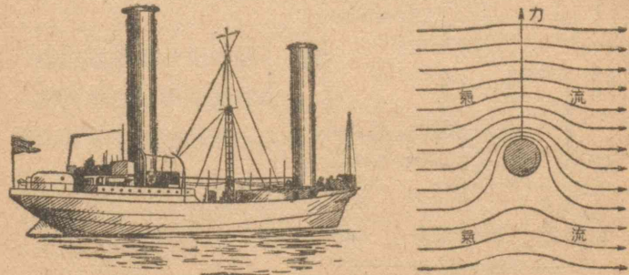
第 88 図 フレットナー船
