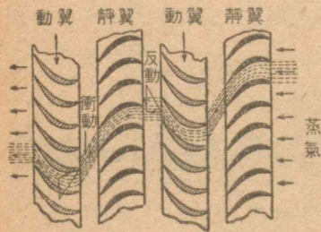
第120図 パーソンズ・タービン
