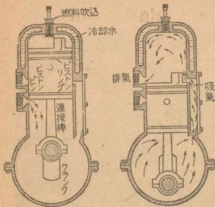
第127図 ジーゼル機関
