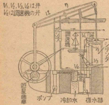
第113図 ワットの復動機関
