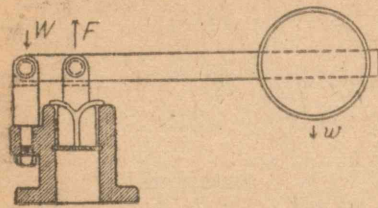
第 26 図 (a) てこ安全弁
