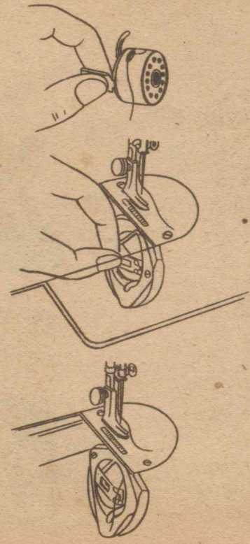
下糸の引き出し方
