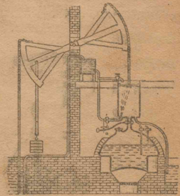
ニュー=コメンの大気圧機関
