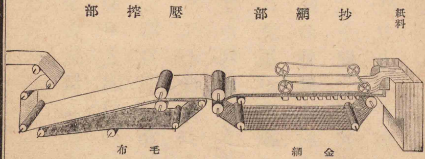
抄紙機
