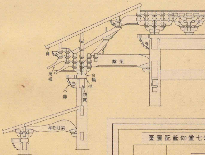
唐様建築手法
