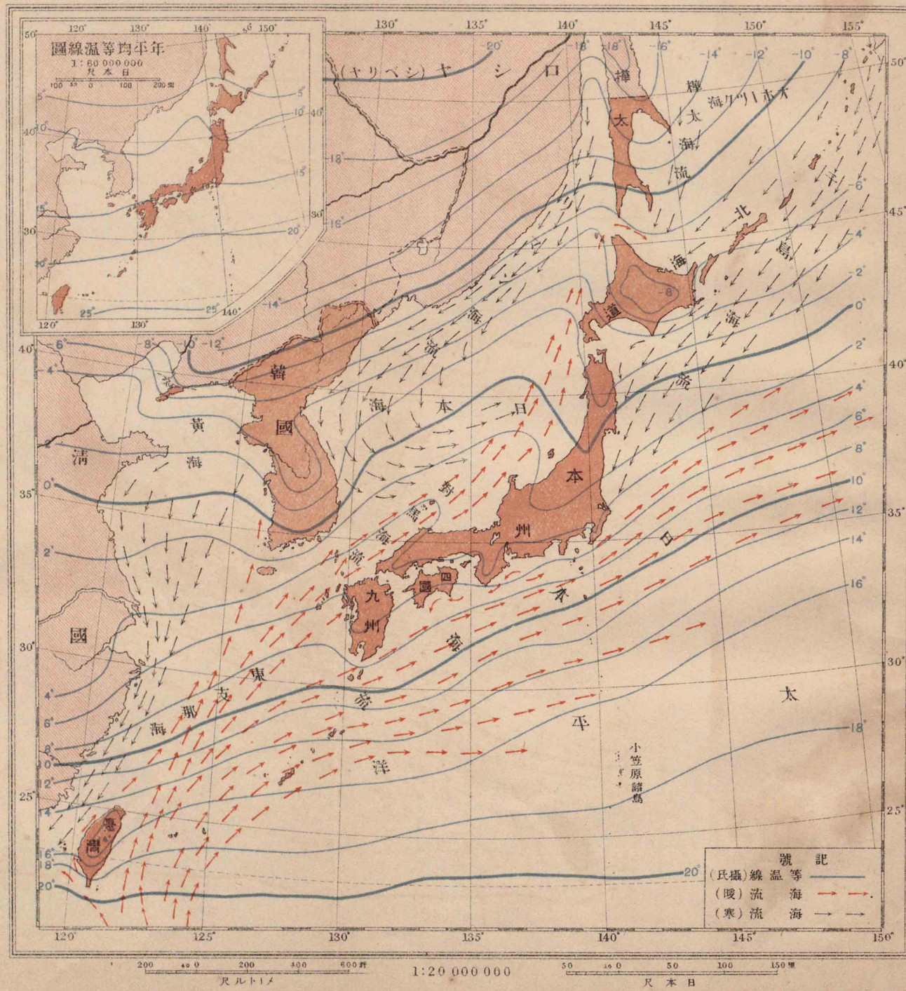
(月二)圖線溫等流海近附本日
