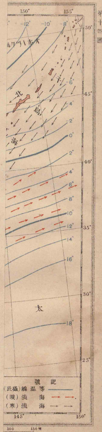
第十四圖 日本附近海流等溫線圖(二月)
