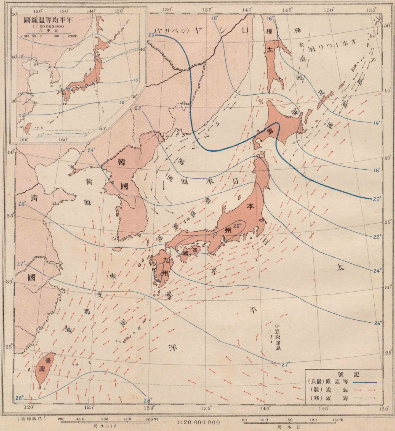
（月八）圖線溫等流海近附本日
