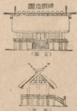
挿繪 皇大神宮宮殿圖。
