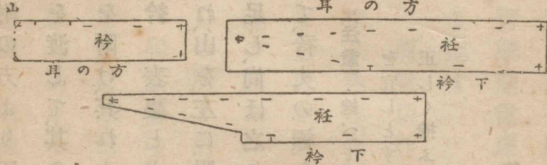
本裁女單衣標附け方
