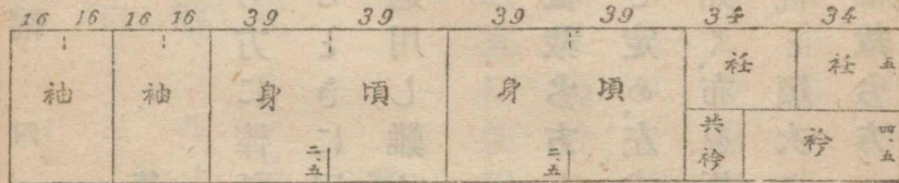
用布の折り方
