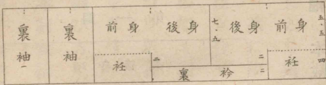
並幅にて四つ身胴裏の裁ち方
