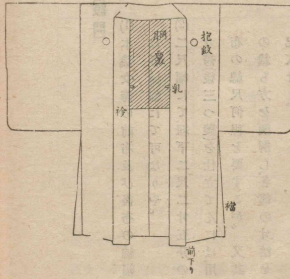
本裁男羽織の圖
