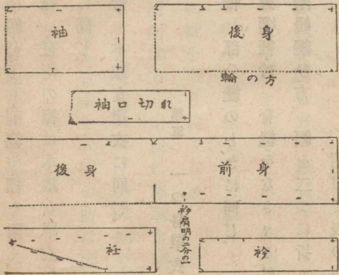
一つ身單衣標附け方
