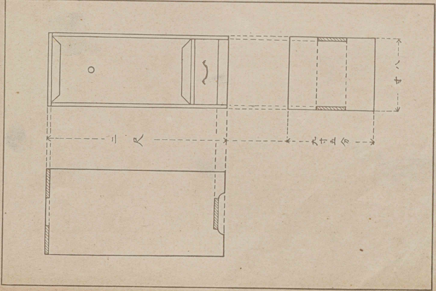
第十三圖 本箱の工作圖
