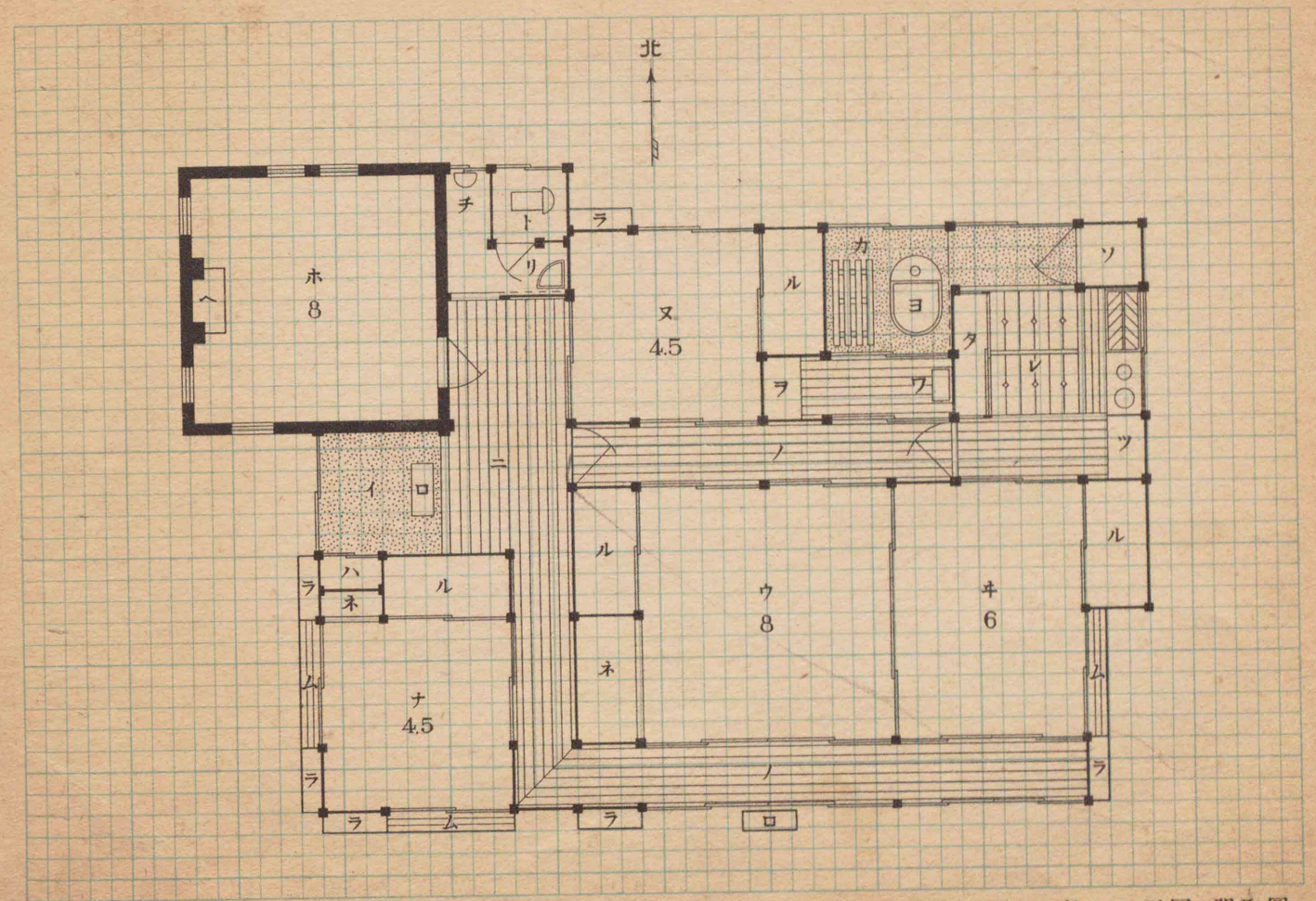
第二十三圖 間取圖
