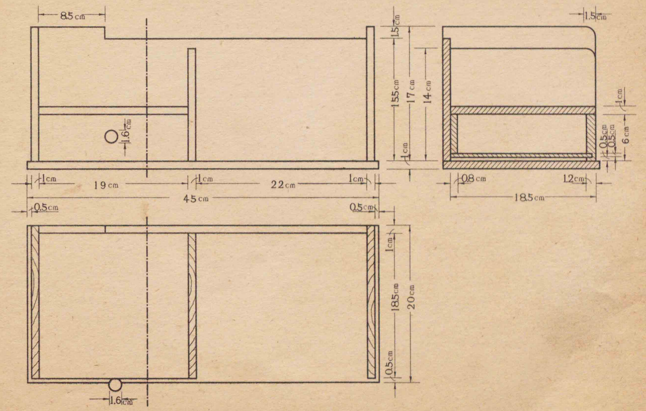
第二圖 本立の製圖
