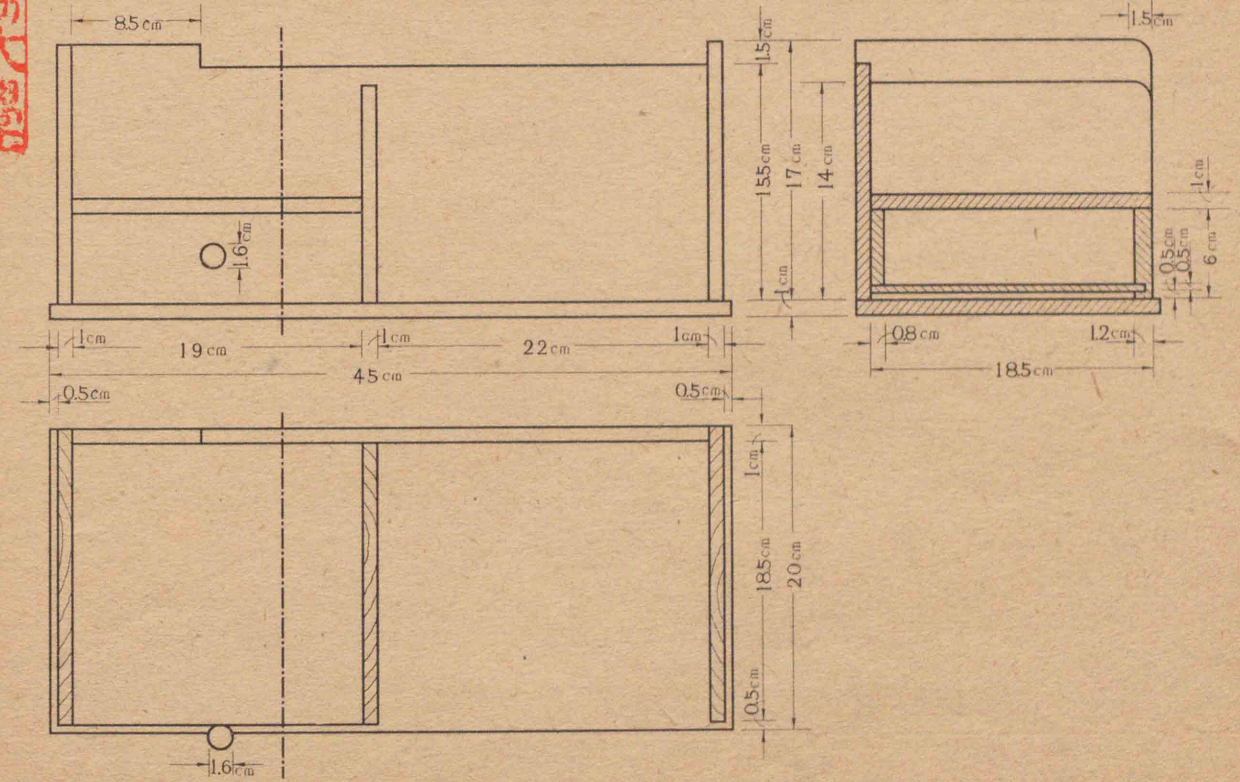
第二圖 本立の製圖
