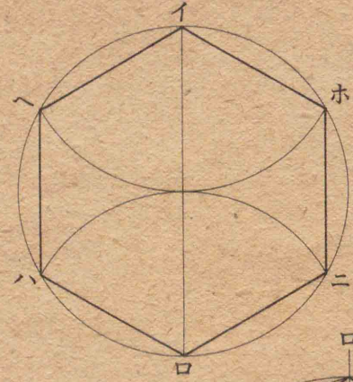
正六角形ノ畫キ方
