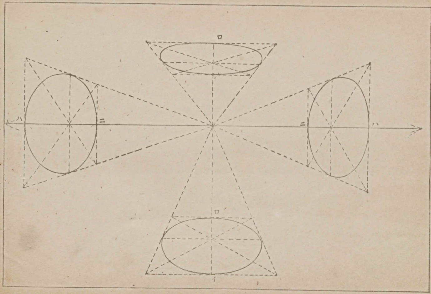
第五圖 圓の透視圖
