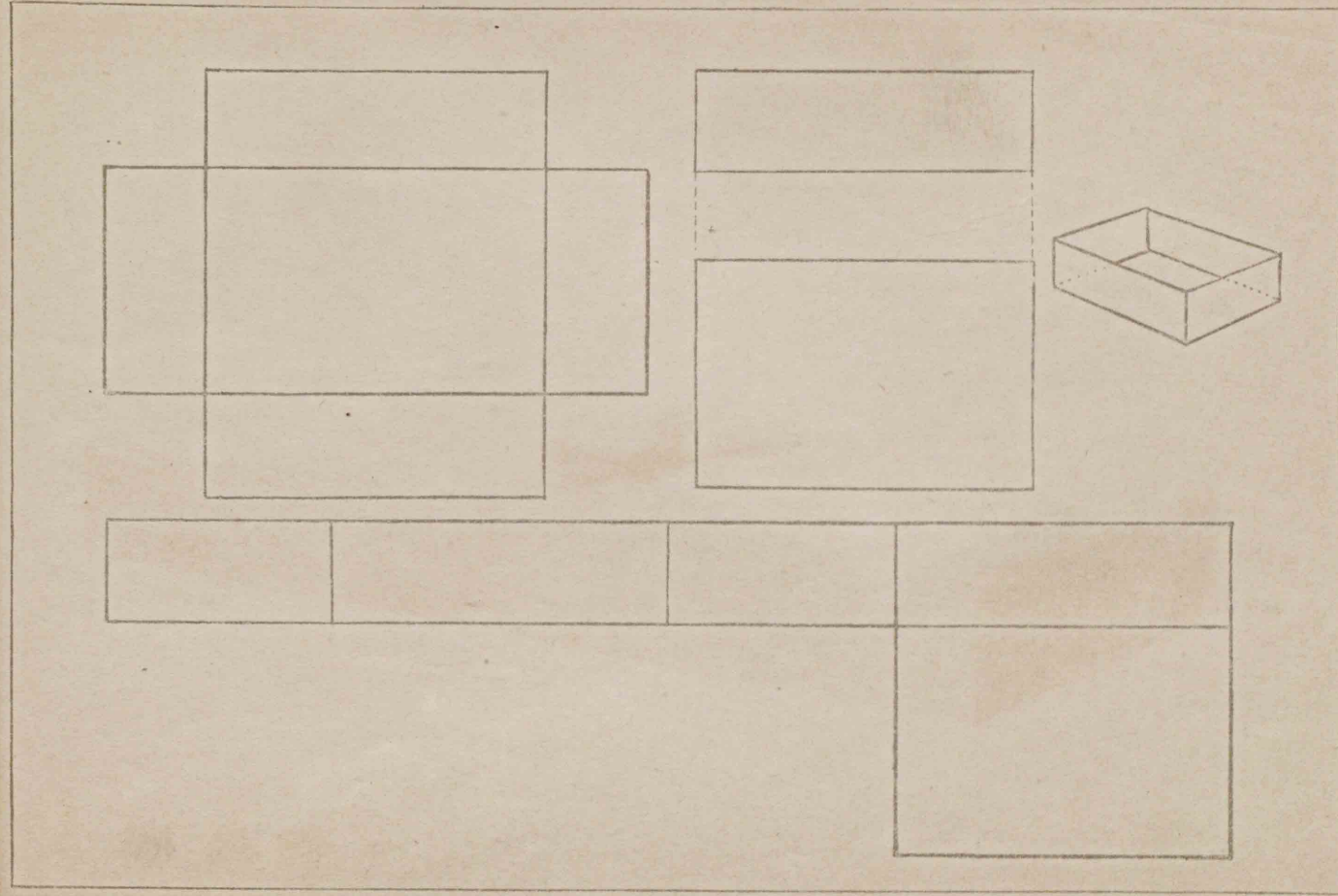
第十九圖 箱の工作圖
