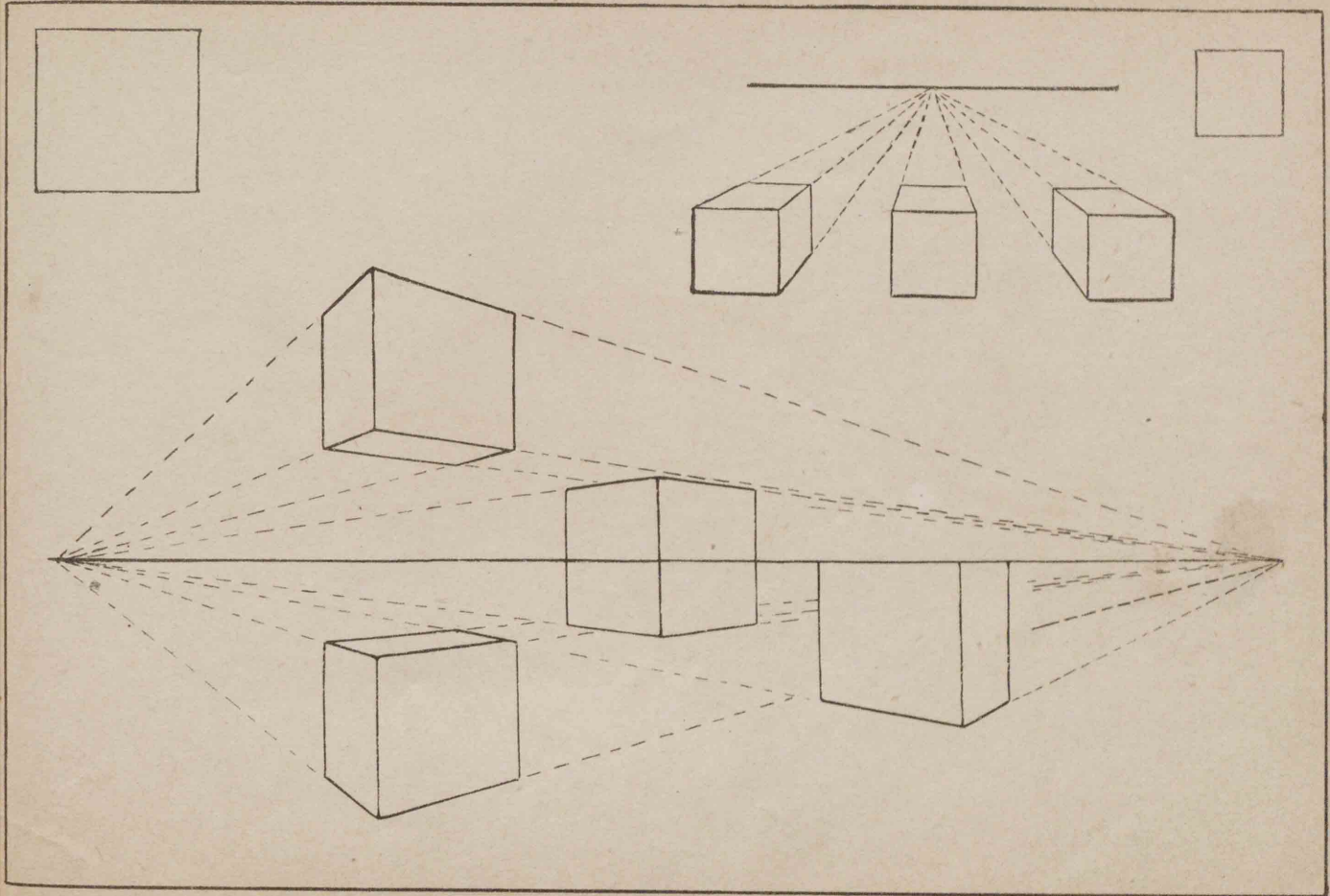
第十圖 立方體の透視圖
