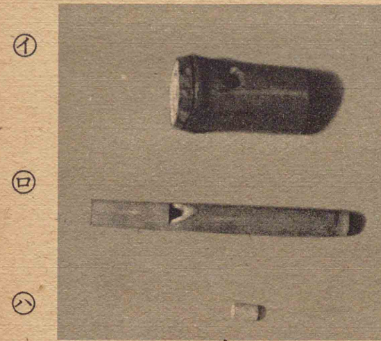
センノアル笛ノ分解圖
