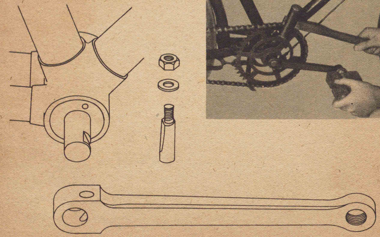
クランクノ分解圖
