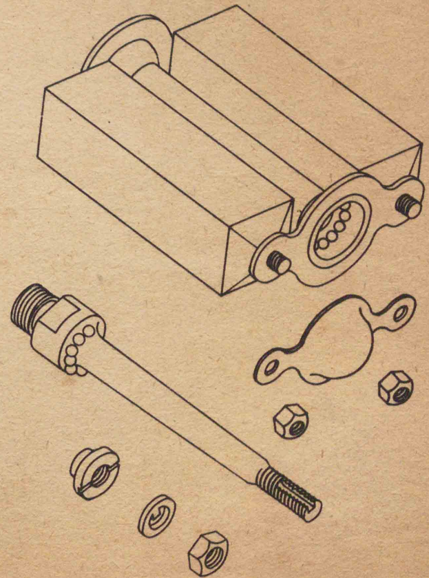
ペダルノ分解圖
