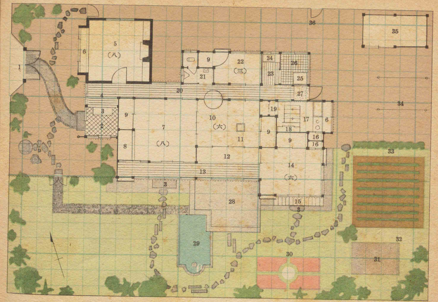
9. 間取圖
